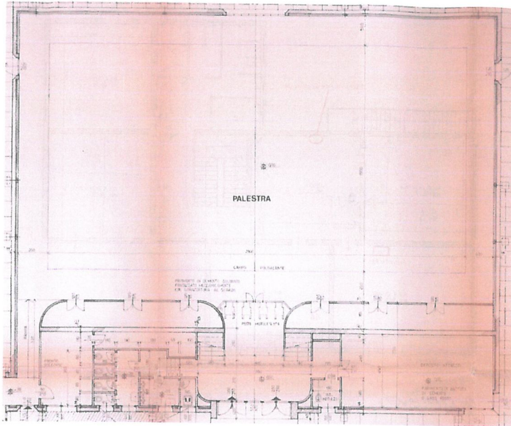
Planimetria PALESTRA
